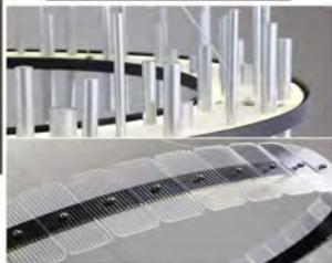
型号: LY100P 光源: LED 材质: 五金 (沙黑+沙银) 规格: (直径*高) \Phi 600^*H370\text{mm} 4000K 48W 价格: ¥7299
